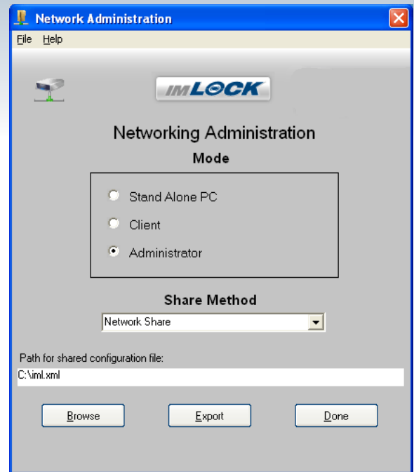
IM Lock Network Administration
